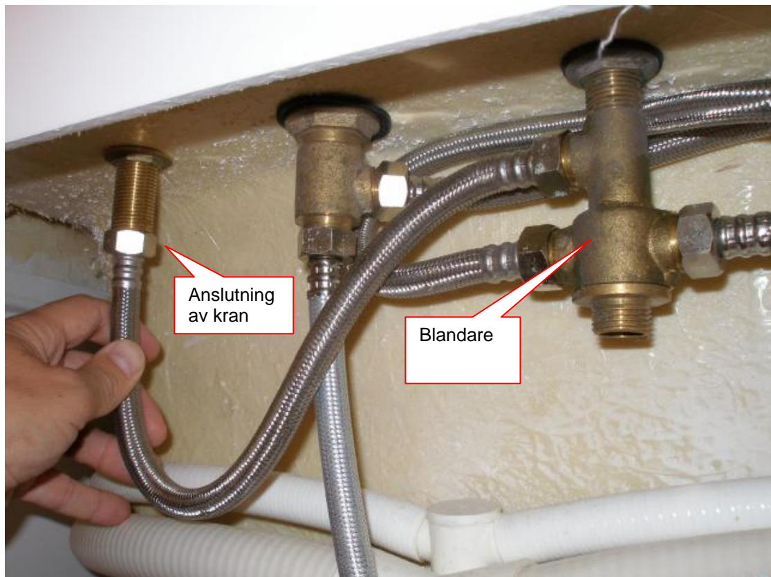
Bild 4 Anslut kranen till blandaren
