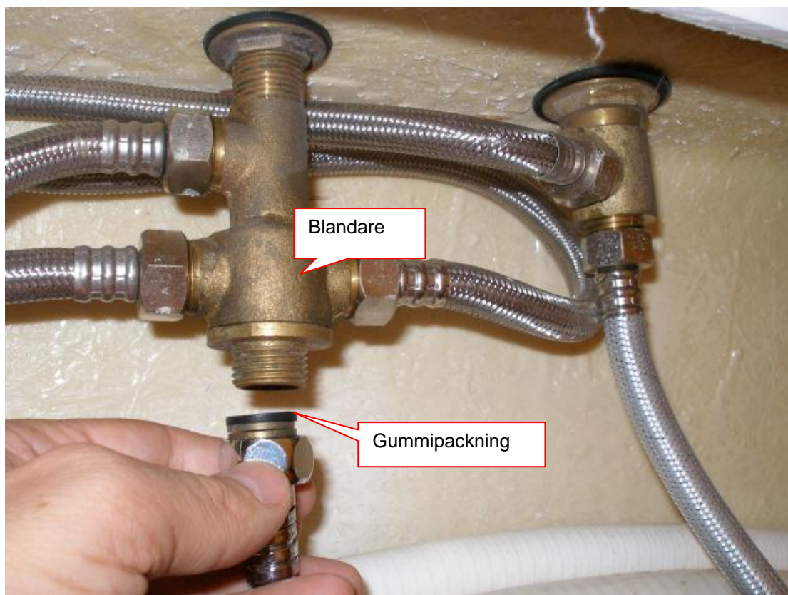
Bild 7 Anslut duschslang till Blandaren
